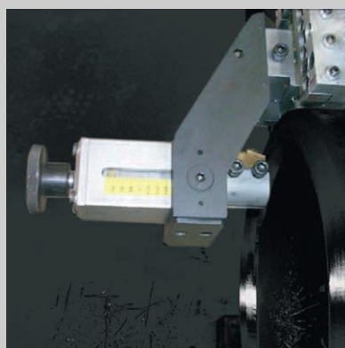
Prípravok pre opracovanie vnút.priemeru použiteľný pre všetky modely. Bezpečné upnutie na nožový suport.
