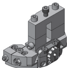
Predĺžený nožový suport s hviezd. kolieskom
